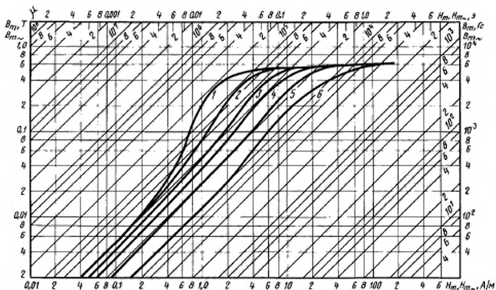
Кривые намагничивания сплава марки 80HXC толщиной 0,1 мм для частот: 1 — 0 Гц; 2 — 400 Гц; 3 — 1000 Гц; 4 — 2000 Гц; 5 — 4000 Гц; 6 — 10000 Гц
