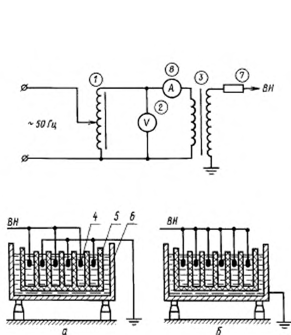
а — схема подключения электродов к источнику высокого напряжения при испытании перегородок моноблока; б — схема подключения электродов к источнику высокого напряжения при испытании корпуса моноблока. 1 — автотрансформатор регулировочный; 2 — вольтметр; 3 — высоковольтный трансформатор — источник высокого напряжения; 4 — электроды; 5 — моноблок; 6 — резервуар; 7 — защитное сопротивление; 8 — амперметр.
