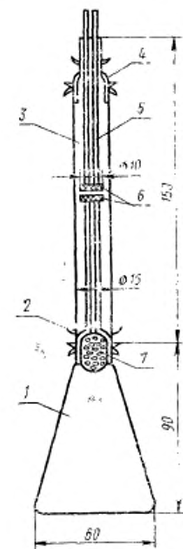
1—колба; 2—пробка; 3—кожух стеклянный; 4—пробка; 5—труб- ка; 6—шланг; 7—тампон ватный
