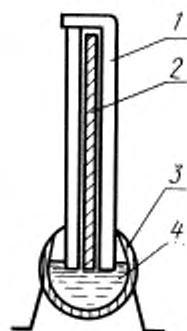
Камера для восходящей хроматографии
