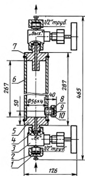
Пробоотборник ПГО-400
