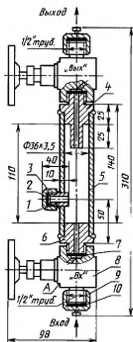
Пробоотборник ПГО-50
