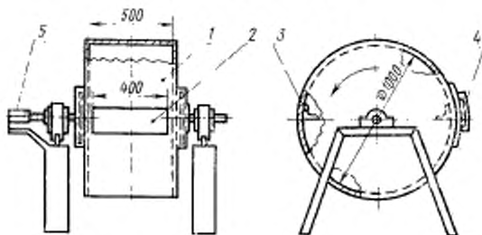
1—барабан; 2—загрузочный люк; 3—уголки; 4—крышка люка; 5—счетчик оборотов
