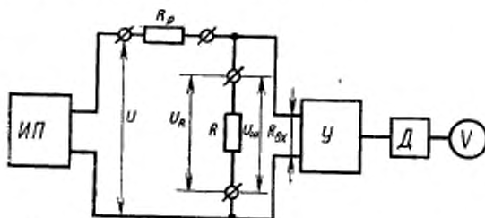
ИП—источник питания постоянного тока; У—усилитель напряжения; Д—квадратный детектор; V—вольтметр; R_p —разделительный резистор; R—испытуемый резистор
