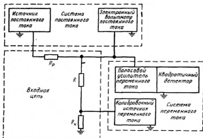
R_p — разделительный резистор; R — проверяемый резистор; R_k — калибровочный резистор
