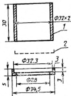
1—трубка, 2—фильтр; 3—зажимное кольцо
