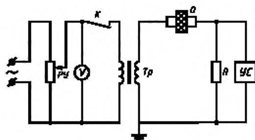
Тр — высоковольтный испытательный трансформатор; R — резистор; РУ — регулятор напряжения; О — образец с электродами; V — вольтметр для измерения напряжения пробоя; ВУ — выпрямительное устройство; C — конденсатор; УС — устройство сигнализации о наступлении пробоя; К — контакт устройства сигнализации, отключающий первичную цепь трансформатора в момент пробоя образца
