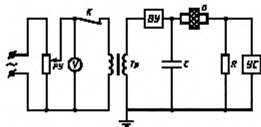
Тр — высоковольтный испытательный трансформатор; R — резистор; РУ — регулятор напряжения; О — образец с электродами; V — вольтметр для измерения напряжения пробоя; УС — устройство сигнализации о наступлении пробоя; К — контакт устройства сигнализации, отключающий первичную цепь трансформатора в момент пробоя образца
