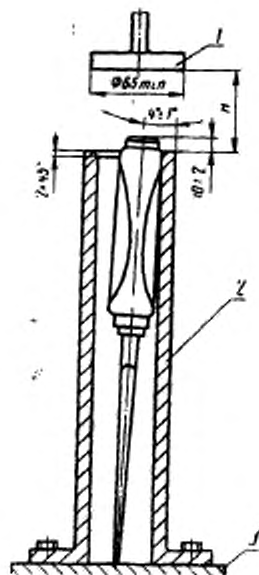
1—гира, обработанная до 61,6...67 HRC 2 ; 2—патрон; 3—основание, обработанное не менее чем до 65 HRC 2
