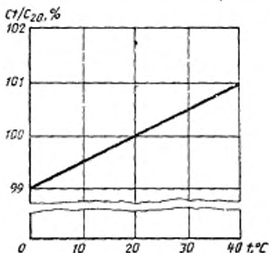
График зависимости емкости от температуры
