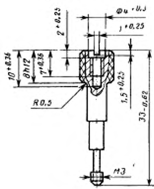
Черт. 24 Крепежный винт
