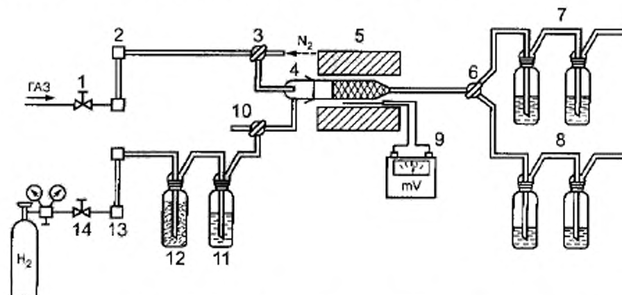
1, 14 — игольчатые вентили; 2, 13 — реометры; 2, 6, 10 — трехходовые краны; 4 — кварцевая трубка; 5 — электрическая печь; 7 — склянки с дистиллированной водой; 8 — склянки с поглотительным раствором; 9 — милливольтметр; 11 — склянка — увлажнитель водорода; 12 — склянка с активированным углем
