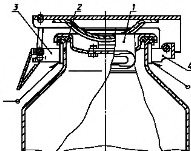
1 — верхний обруч; 2 — горловина; 3 — передний кронштейн; 4 — задний кронштейн
