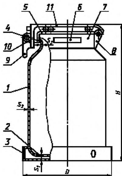
1 — корпус; 2 — днище; 3 — опорный обрuch; 4 — горловина; 5 — крышка; 6 — ручка; 7 — верхний обрuch (для флаг типа ФА); 8 — задний кронштейн; 9 — затвор; 10 — передний кронштейн; 11 — прижим
