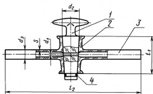
Краны типов K1X и K1X КШ
