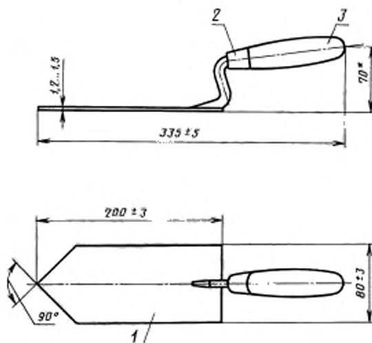
Лопатка типа ЛК
