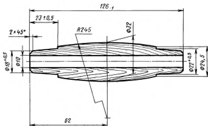
Ручка для кельм типов КБ и КП
