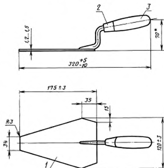
Лопатка типа ЛП
