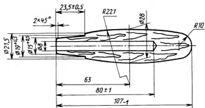
Ручка для отрезки
