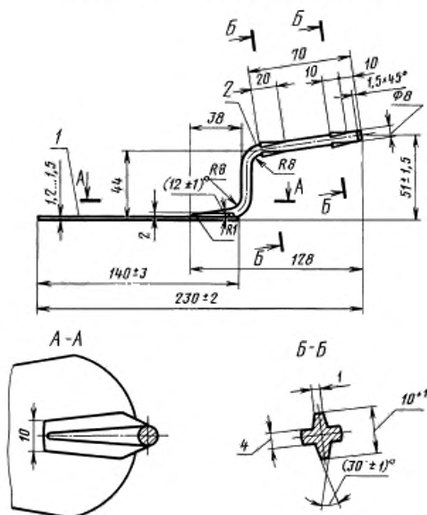
Полотно с кронштейном отрезки типа ОШ
