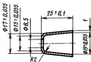
Колпачок для отрезки
