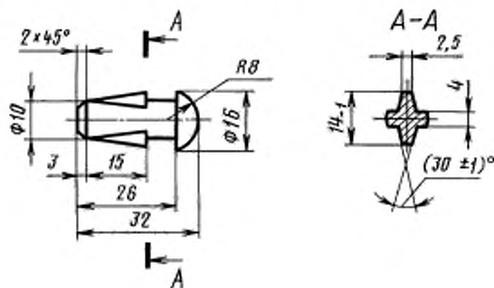
Грибок для кельм типов КБ и КП
