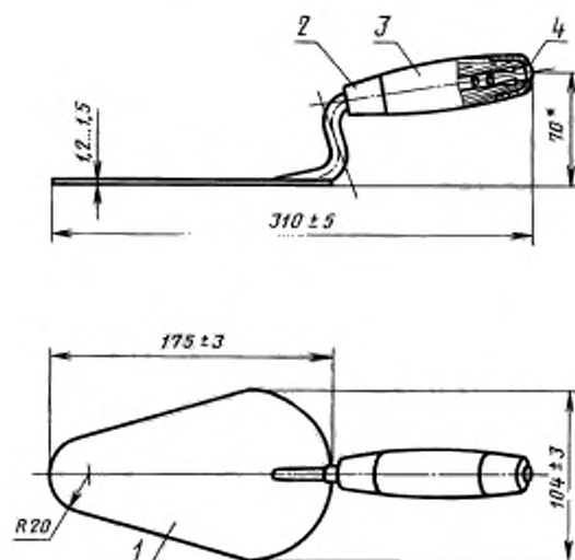
Кельма типа КП
