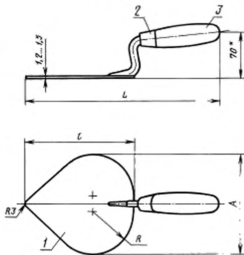
Кельма типа КШ
