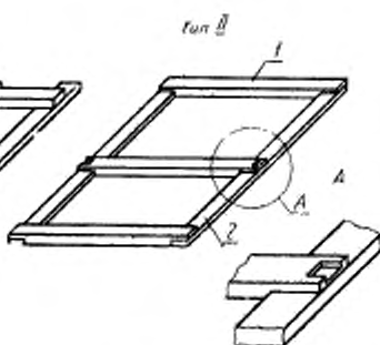
1—поперечная планка; 2—продольная планка
