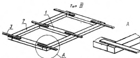
1—поперечная планка; 2—продольная планка; 3—стальная лента
