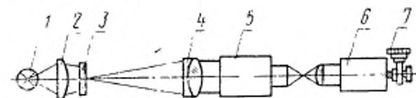
1—источник света; 2—конденсор; 3—мира; 4—объектив коллиматора; 5—анаморфотный кино съемочный блок или насадка с объективом; 6—микроскоп; 7—окулярный микрометр
