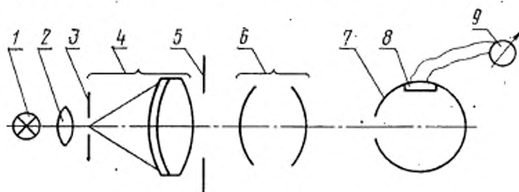
1—источник света; 2—конденсор; 3—точечное отверстие; 4—коллиматор; 5—ирисовая диафрагма; 6—испытуемая система; 7—фотометрический шар; 8—фотоприемник; 9—регистрационный прибор
