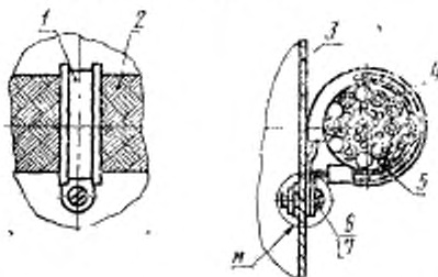
М — место металлизации; 1 — хомут зажимной с обкладкой; 2 — экран жгута; 3 — кронштейн; 4 — жгут; 5 — медная лента; 6 — винт; 7 — гайка
