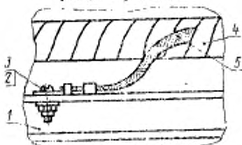
1 — профиль; 2 — винт; 3 — гайка; 4 — жгут; 5 — перемычка
