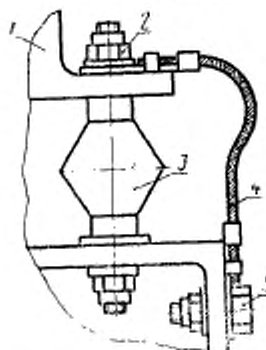
1 — прибор; 2 — гайка; 3 — амортизатор; 4 — неразъемная перемычка типа А по ГОСТ 18707; 5 — болт
