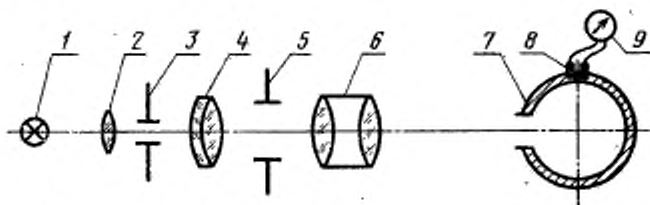
1—источник света; 2—конденсор; 3—коллиматорная диафрагма; 4—объектив калибратора; 5—диафрагма с калиброванным отверстием; 6—испытуемый объектив; 7—фотометрический шар; 8—фотоприемник; 9—отсчетное устройство
