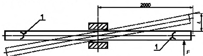
1 — посадочное место; L — отклонение корпуса относительно продольной оси; F — горизонтальная нагрузка (695 \pm 5) Н
