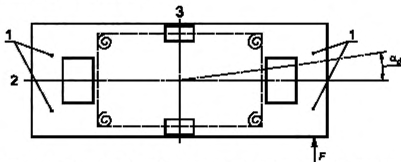
1 — посадочное место; 2 — продольная ось; 3 — поперечная ось; \alpha_d — угол отклонения корпуса относительно продольной оси; F — горизонтальная нагрузка (695 \pm 5) Н
