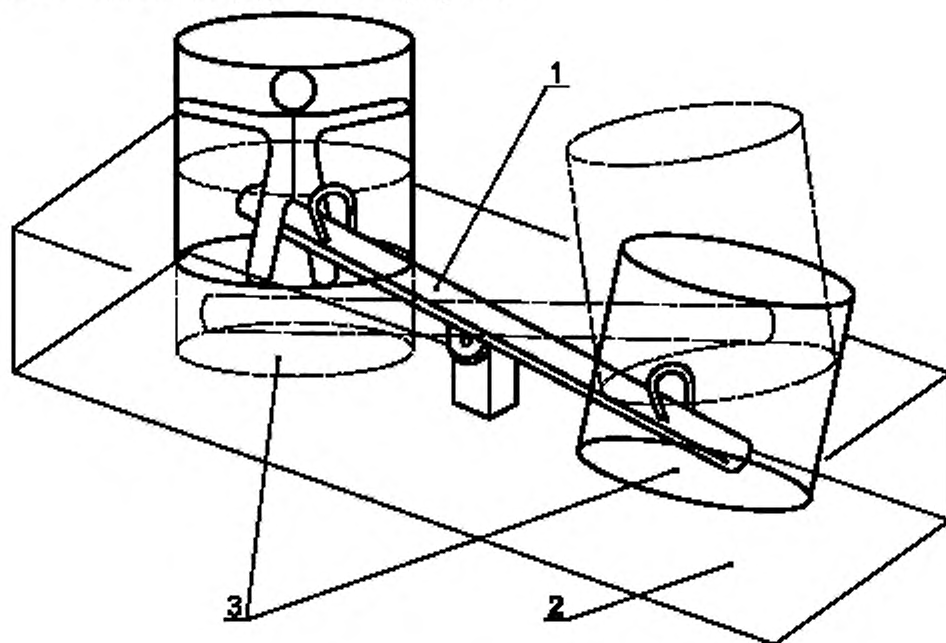
1 — качалка; 2 — зона приземления качалки; 3 — зона безопасности
