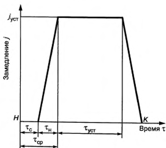
Тормозная диаграмма (схема)
