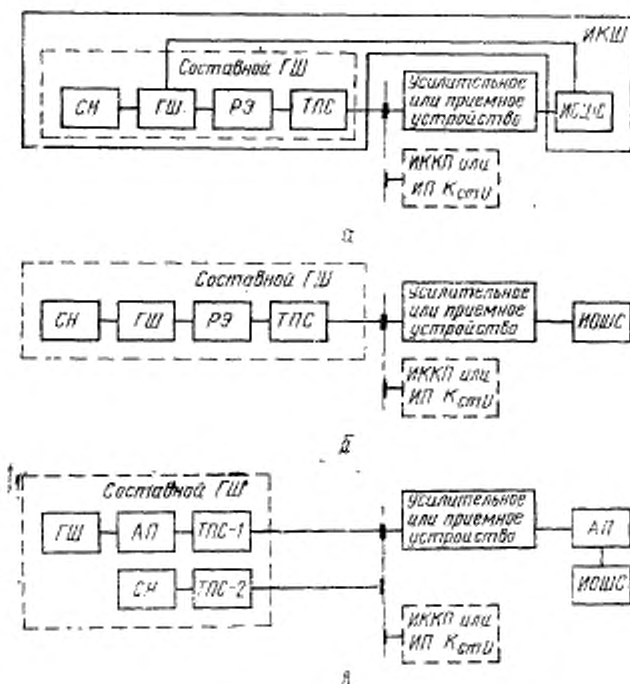
а — схема стенда для измерения коэффициента шума с использованием промодулированного генератора шума (ГШ); б — то же, методом двух отсчетов; в — схема стенда для прецизионных измерений с использованием аттестованного поляризационного аттенюатора (АП)
