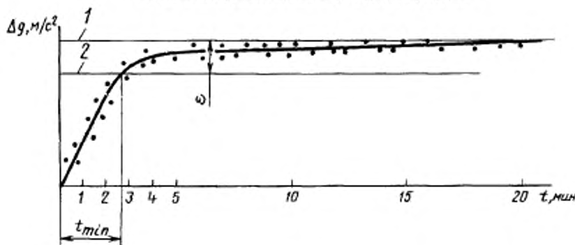
Определение длительности переходного процесса
