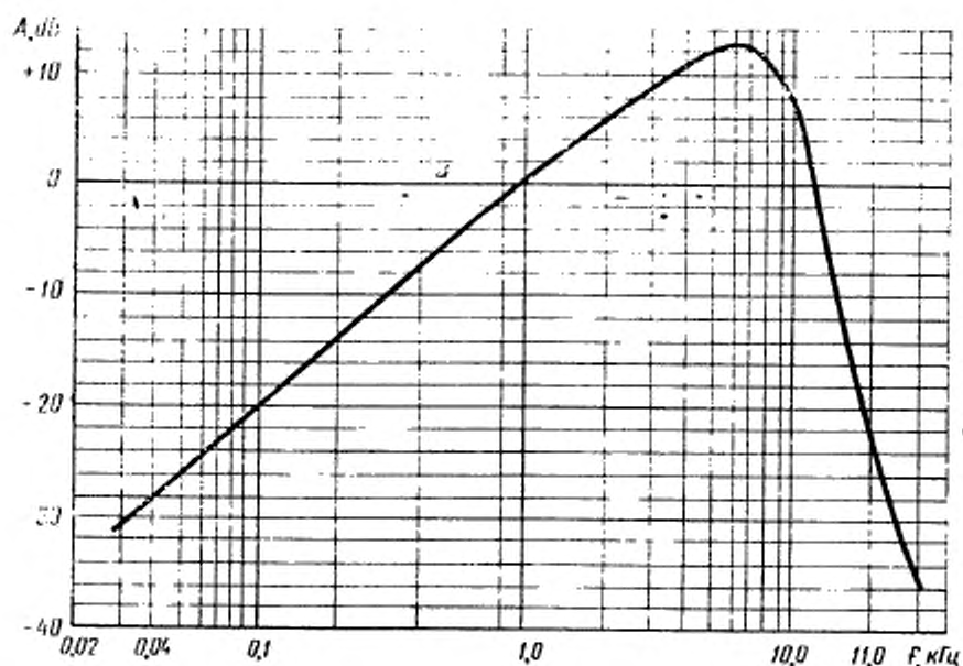
Амплитудно-частотная характеристика псофометрического фильтра
