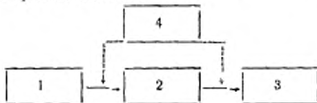
1 — исследуемый лазер; 2 — оптическая система; 3 — средство измерений; 4 — средство юстировки
