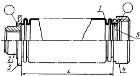
1—сильфон; 2—втулка; 3—кольцо; 4—втулка; 5—кольцо
