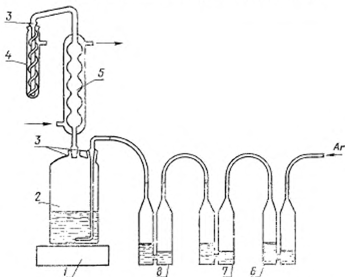
1—электролитная; 2—сосуд реакционный с восстановительной смесью; 3—шпильки; 4—приемник с щелочным раствором гидросилимина и трилона Б (спиральная кварцевая засадка, приваренная к наружной стороне выходной трубки обратного холодильника); 5—обратный холодильник; 6, 7—барботер с 25 %-ным раствором пирогазола в 25 %-ном растворе едкого кали; 8—барботер с дистиллированной водой.
