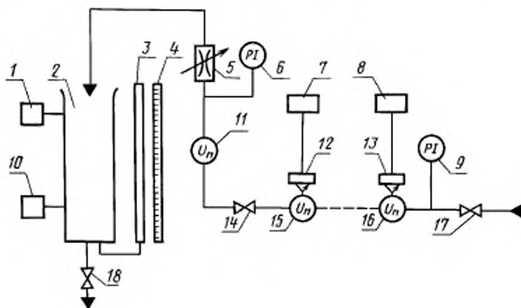
Принципиальная схема измерительной части установки с оптоэлектронным узлом съема сигналов для поверки счетчиков и одной меры вместимости
