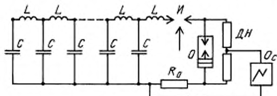
C, L — емкости и индуктивности генератора импульсов тока большой длительности соответственно; I — управляемый искровой промежуток; R_g — шунт для измерения тока; O — испытуемый образец или разрядное сопротивление; DH — делитель напряжения; Oc — осциллограф
