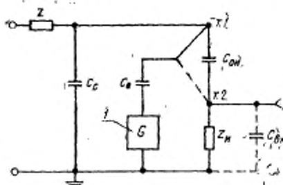
Схема соединений при эквивалентной градуировке
