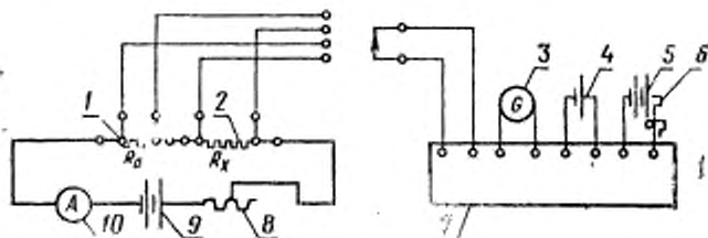
1—набор образцовых сопротивлений класса 0,01 (эталонных); 2—исследуемое сопротивление; 3—гальванометр чувствительностью порядка 1 \cdot 10^{-9} А/дел.; 4—порционный элемент Вестона; 5—источник постоянного тока; 6—реостат; 7—потенциометр постоянного тока или мост Томсона; 8—реостат; 9—источник постоянного тока; 10—амперметр постоянного тока класса 0,5.
