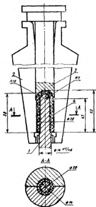
1—ротор; 2—матрица; 3—пуансон; 4—образец Черт. 2
