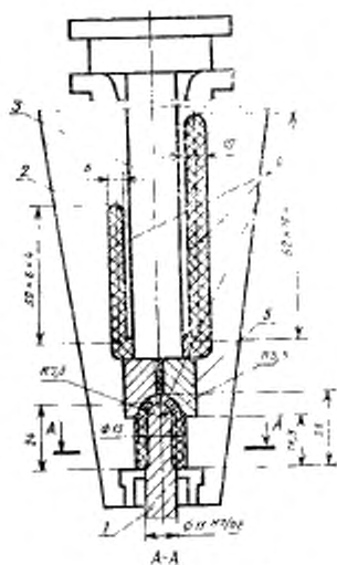
Пресс-форма 3
