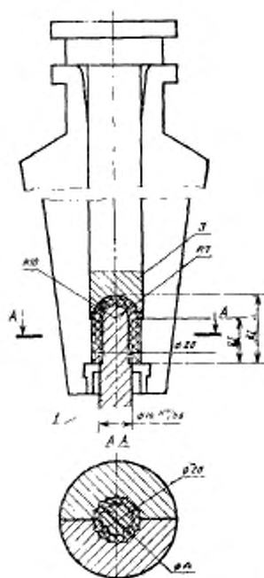
Пресс-форма 2
