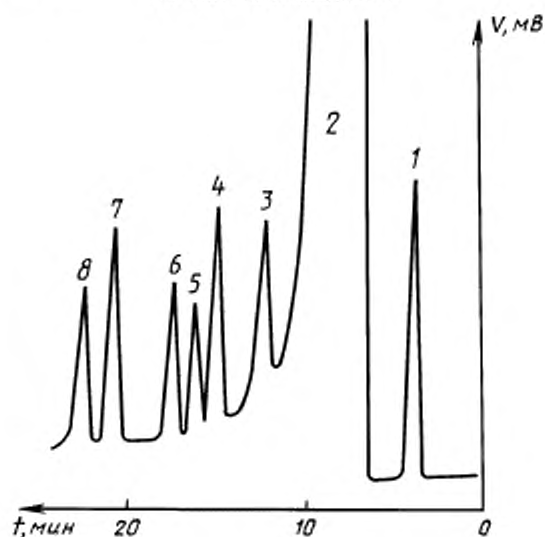
Типовая хроматограмма искусственной смеси четыреххлористого углерода и хлорорганических примесей на колонке с насадкой II
