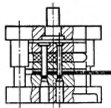
Штамп последовательного действия для пробивки и вырубки
