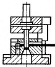
Штамп простого действия для вырубки
