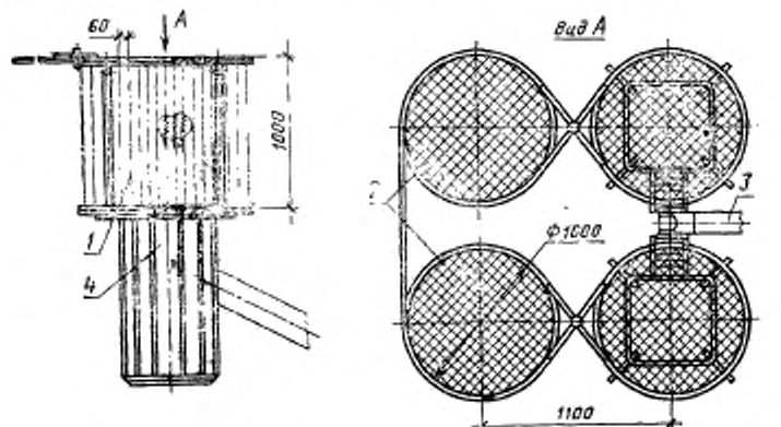
1 — основной экран; 2 — дополнительный экран; 3 — стрела гидродъемника; 4 — дюлька гидродъемника
