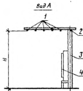
1 — канаты; 2 — дополнительный канат; 3 — конструкция для крепления экрана; 4 — шкафы
