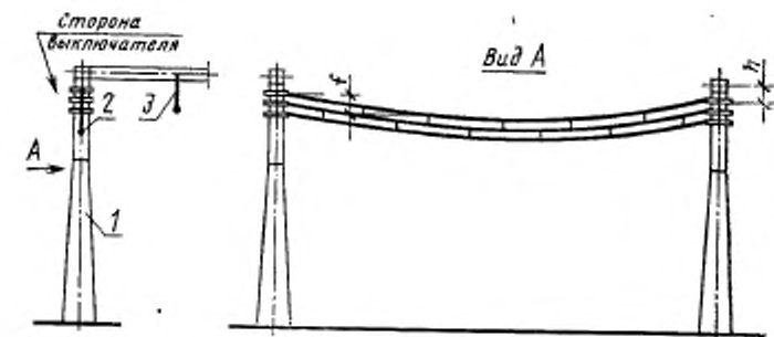
1 — портал сборных шин; 2 — канаты экрана; 3 — провода системы шин, фаза А (С); f — провес экрана
