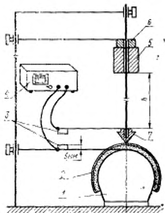
1—модель головы; 2—шлем; 3—электроконтакты; 4—электроизмерительный прибор; 5—ударник; 6—электромагнит; 7—пробойник Черт. 12
