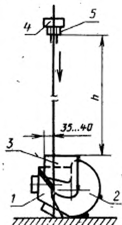
1 — модель головы; 2 — шлем; 3 — экран; 4 — электроударник; 5 — ударник
