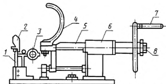
1 — силовизмерительная пружина; 2 — передний держатель; 3 — индикатор часового типа; 4 — задний держатель; 5 — поджимной шток; 6 — подшипник; 7 — ручной привод; 8 — ограничительная пробка
