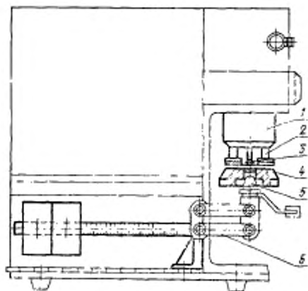
1 — истирающая головка; 2 — бегунок; 3 — устройство для натяжения испытуемой или абразивной ткани; 4 — вальцы; 5 — опора вальцев; 6 — рычажно-грузовая система для создания нормального давления
