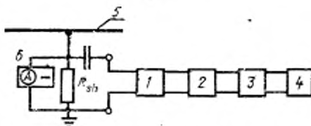
1 — устройство согласования для коэффициента k_f , состоящее из одного резистивно-емкостного звена; 2 — усилитель; 3 — ваттометр; 4 — самопишущий измерительный прибор; 5 — контактный провод; 6 — вольтметр постоянного тока, градуированный в амперах
