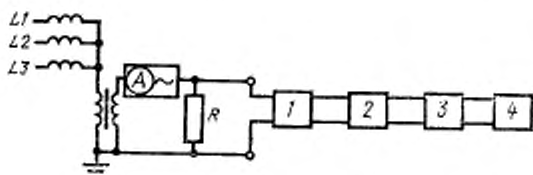
1 — устройство согласования для коэффициента k_f , 2 — усилитель; 3 — ваттометр, 4 — самопишущий измерительный прибор
