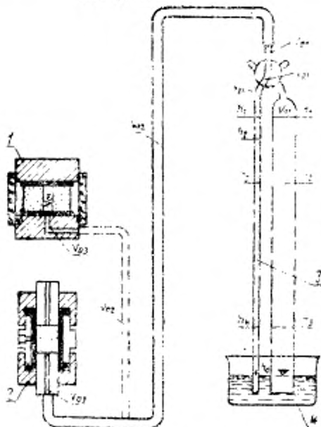
1—кранодержатель радиальный. 2—кранодержатель ливневый; 3—двухрубный пьезометр; 4—сосуд для жидкости
