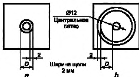
Рисунок 13 — Размеры мишеней
