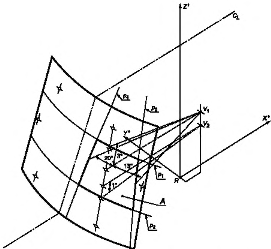
C_c — след продольного среднего сечения ТС; p_i — след соответствующей плоскости
