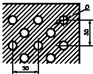
Рисунок 10 — Увеличенная деталь
