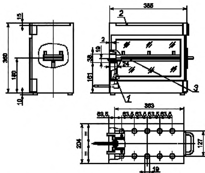
1 — газовая горелка; 2 — вентиляционная щель; 3 — образец для испытаний
