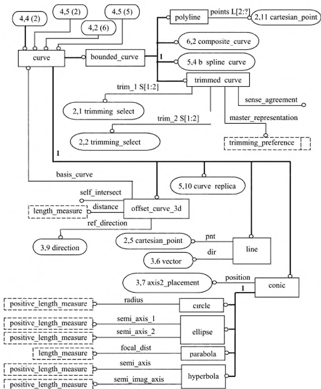
Рисунок С.4 — alc_geometrically_bounded_wireframe — EXPRESS-G диаграмма 4 из 6
