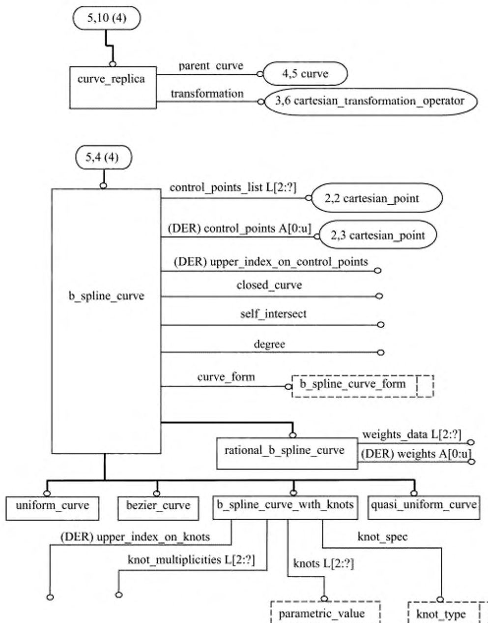
Рисунок С.5 — alc_geometrically_bounded_wireframe — EXPRESS-G диаграмма 5 из 6
