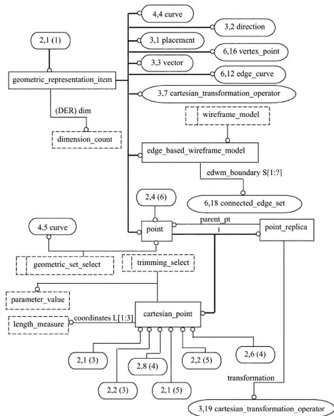
Рисунок C.2 — alc_edge_based_wireframe — EXPRESS-G диаграмма 2 из 6
