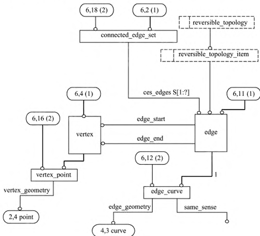
Рисунок С.6 — alc_edge_based_wireframe — EXPRESS-G диаграмма 6 из 6
