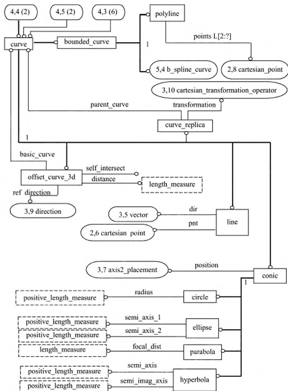
Рисунок С.4 — a1c_edge_based_wireframe — EXPRESS-G диаграмма 4 из 6
