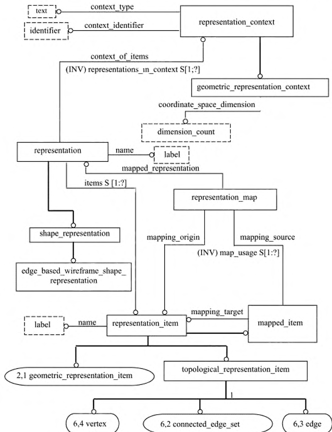
Рисунок С.1 — alic_edge_based_wireframe — EXPRESS-G диаграмма 1 из 6
