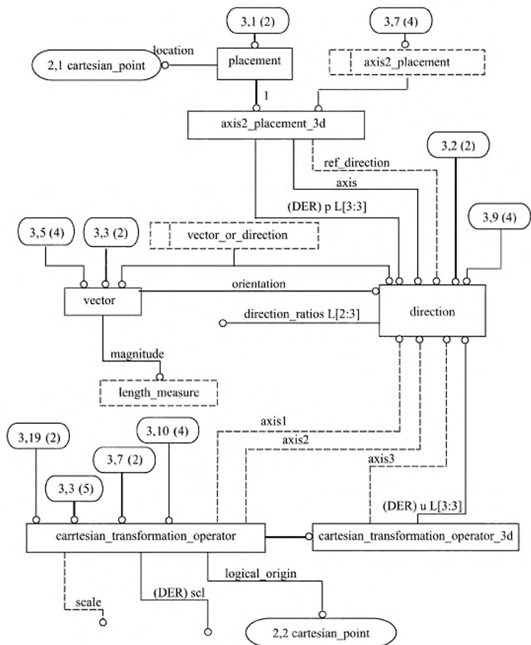
Рисунок С.3 — alic_edge_based_wireframe — EXPRESS-G диаграмма 3 из 6
