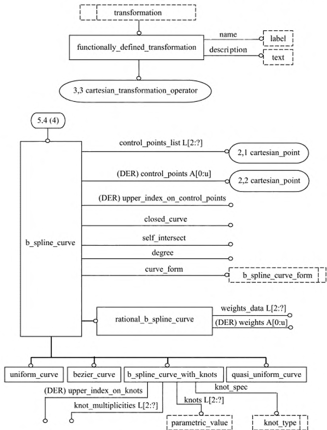
Рисунок С.5 — alc_edge_based_wireframe — EXPRESS-G диаграмма 5 из 6
