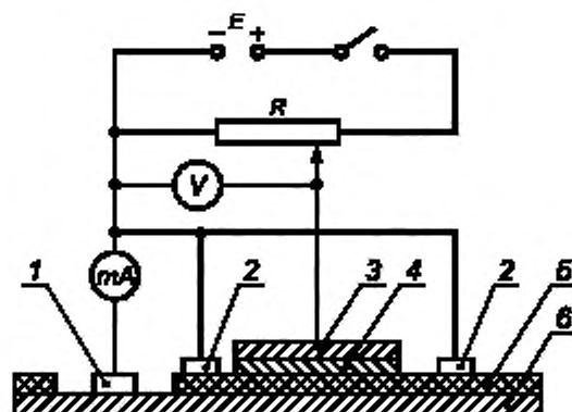
1 — контакт с трубой; 2 — экранирующие кольцевые электроды-бандаж; 3 — кольцевой электрод-бандаж; 4 — тканевое полотно; 5 — изоляционное покрытие трубы; 6 — стенка трубы; E — источник постоянного тока; R — потенциометр; V — высокоомный вольтметр; mA — миллиамперметр
