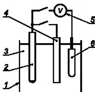
1 — емкость; 2 — испытуемый образец; 3 — электролит; 4 — магневый анод; 5 — вольтметр; 6 — электрод сравнения
