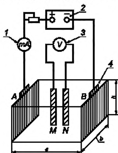
1 — миллиамперметр; 2 — источник тока; 3 — вольтметр; 4 — измерительная ячейка размерами a , b ; h (см. А.2.2); А и В — внешние электроды; М и N — внутренние электроды
