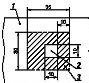
1 — испытываемое покрытие; 2 — образец покрытия для сдвига; 3 — площадь без покрытия
