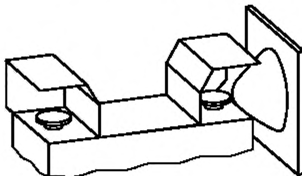
Рисунок А.6 — Применение испытательного конуса
