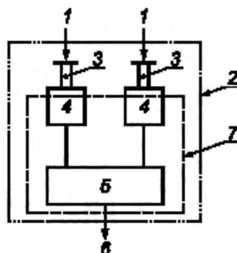
1 — входной сигнал; 2 — двуручное устройство управления; 3 — исполнительное устройство управления; 4 — преобразователь сигналов; 5 — устройство для обработки сигналов; 6 — выходной сигнал; 7 — логический блок
