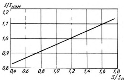
Зависимость тока предохранителя от сечения кабеля
