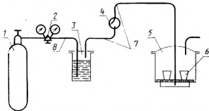
1 - баллон с воздухом; 2 - редуктор газовой; 3 - склянка; 4 - каплеуловитель, 5 - эксикатор; 6 - тигли фарфоровые; 7, 8 - трубки соединительные
