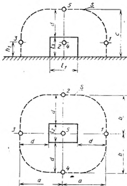
8 — измерительная поверхность; 1—5 — измерительные точки; l_1 ; b_1 ; b — размеры машины; d — измерительное расстояние
