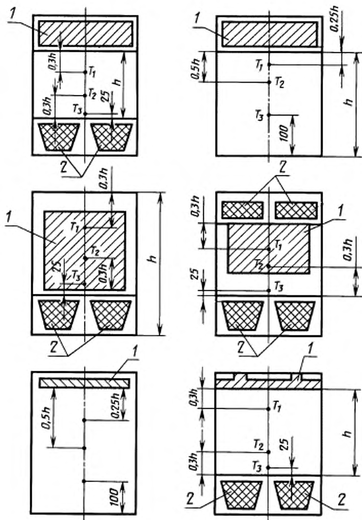
Схемы размещения термомпар при измерении температур в холодильной камере
